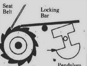
Pendulum
